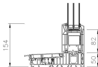
REHAU SYNEGO HS PORTÁL PANORAMA
