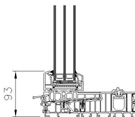
REHAU SYNEGO HS PORTÁL PANORAMA
