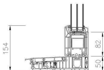
REHAU SYNEGO HS PORTÁL CLASSIC
